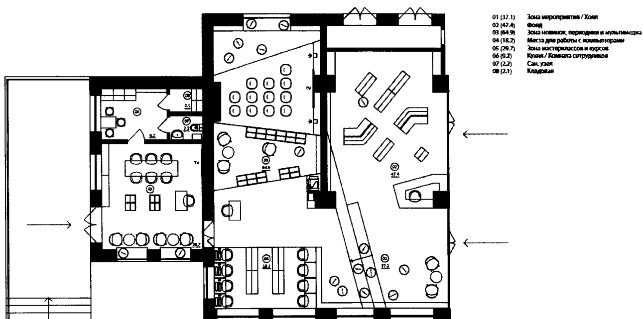
Рисунок 3 План помещений модельной библиотеки
